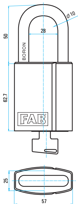
visací zámek FAB DYNAMIC 2413 H
