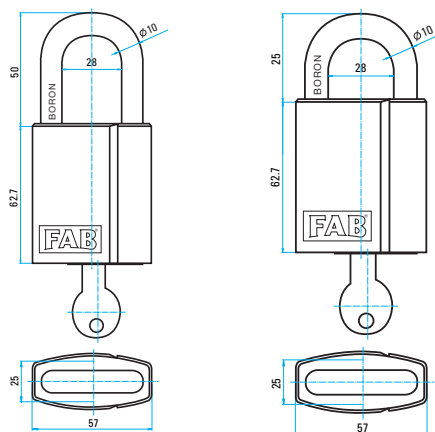
visací zámek FAB 1401 H visací zámek FAB 1400 H
