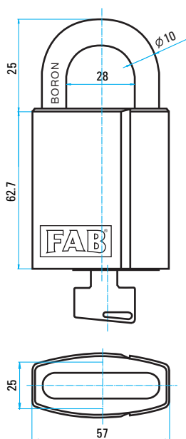
visací zámek FAB DYNAMIC 2414 H
